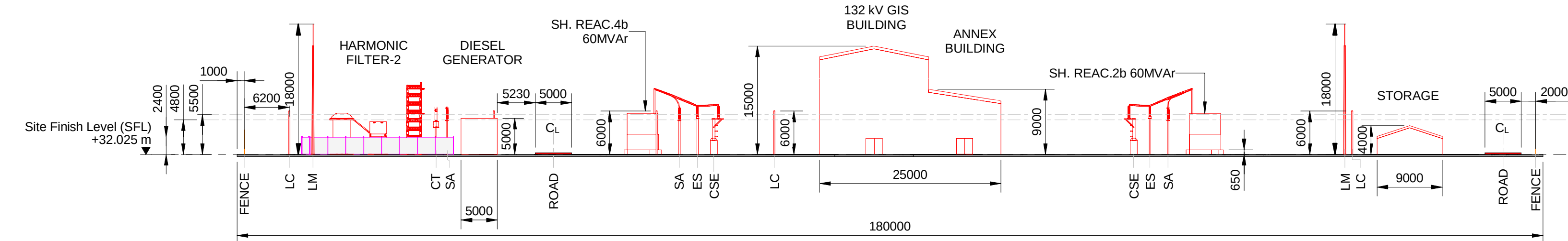
ELEVATION D 1 : 500
